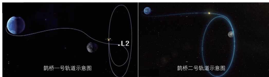
鹊桥一号及鹊桥二号轨道示意图 作者供图
